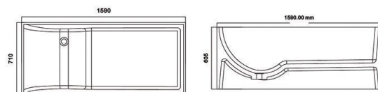
MY005 1590*710*605mm
